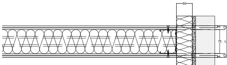
2. Aansluiting aan een massieve wand schaal 1:5
